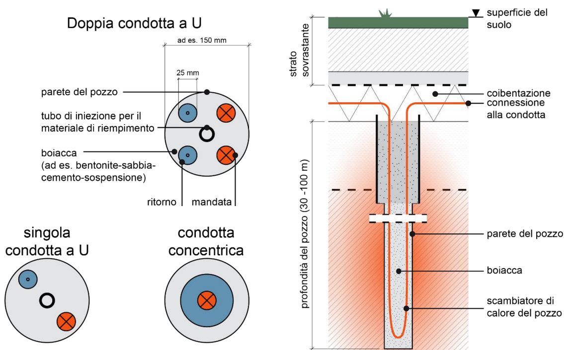
Figura 59: Tipologie comuni e sezione verticale degli scambiatori di calore in pozzo (Fonte: Solites)
