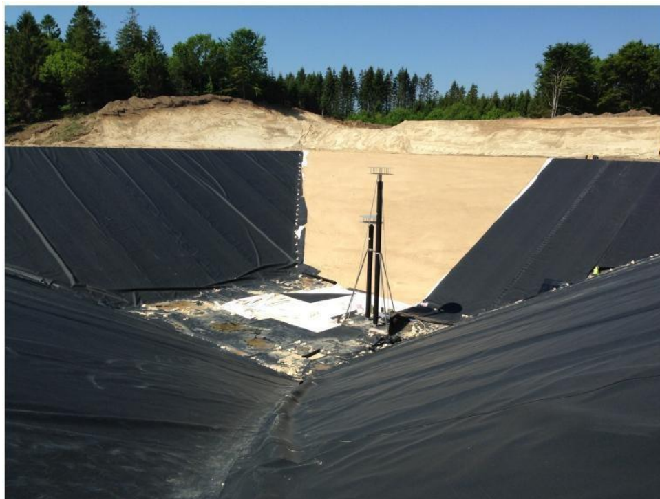
Figura 58: Costruzione del sistema di stoccaggio sotterraneo dell'energia termica SUNSTORE 3 a Dronninglund (Dronninglund Fjernvarme)
