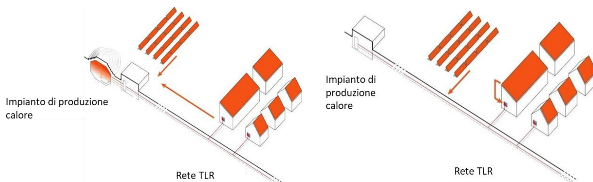
Figura 32: Concetti di integrazione del solare termico nel TLR: i collettori possono fornire calore all'unità di distribuzione centrale (sinistra), oppure, nel caso di impianti decentralizzati ubicati nelle località idonee, sono collegati direttamente con la rete (destra) (Fonti: Solites)
