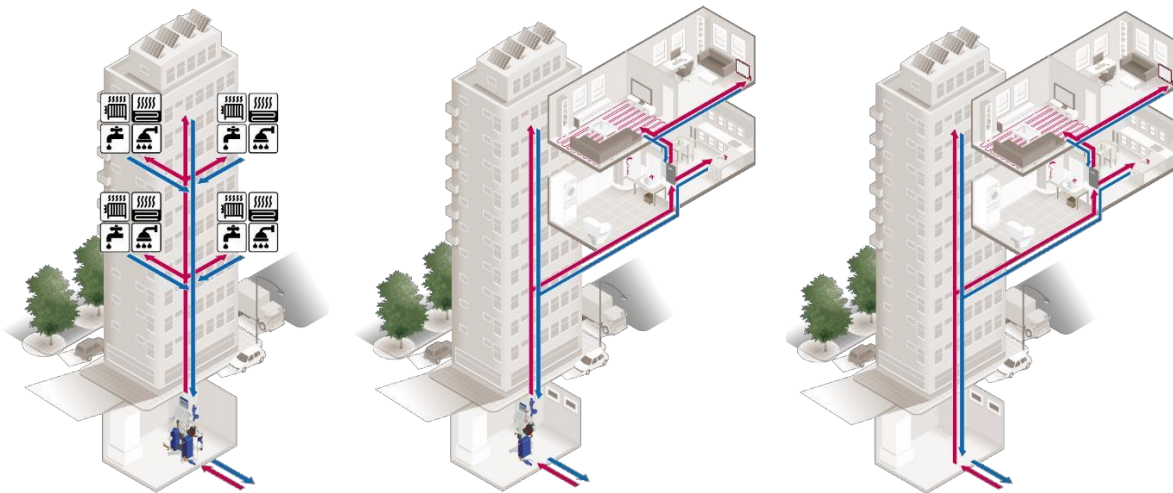
Figura 26: Concetti di collegamento tra unità abitative e teleriscaldamento (Fonte: Alfa Laval / Cetetherm – COOL DH project)
