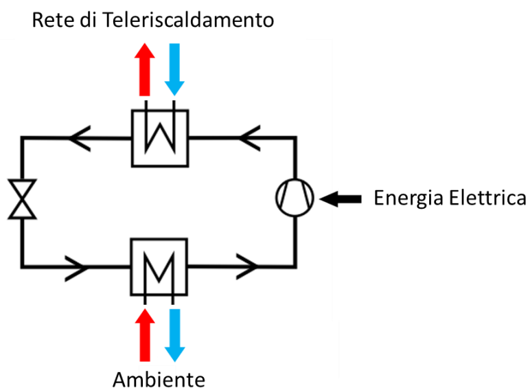
Figura 54: Principio di funzionamento delle pompe di calore a compressore (secondo AGFW, 2017)
