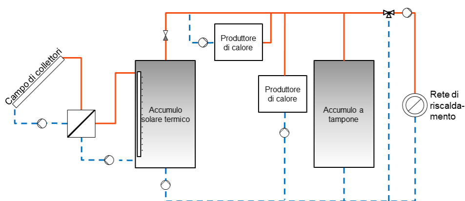
Figura 38: Collegamento in serie dei collettori solari termici alla rete di teleriscaldamento e teleraffreddamento con un sistema di innalzamento della temperatura esterno allo stoccaggio (Fonte: SOLITES)
