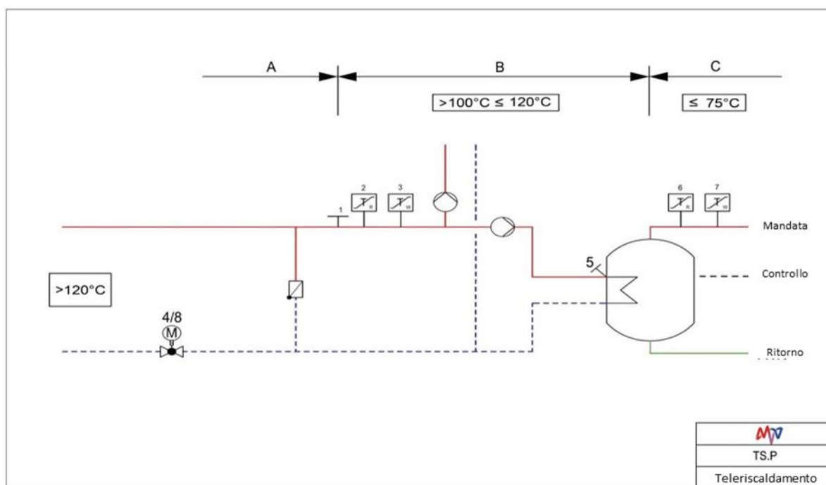
Figura 7: Lo schema di un sistema diretto (Fonte: MVV Netze, 2015)
