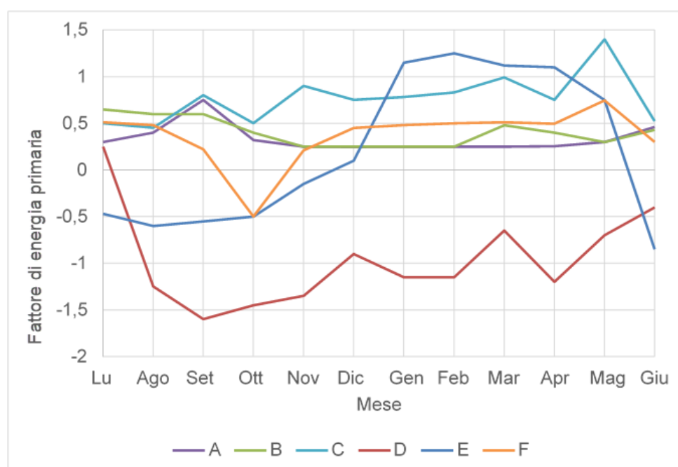
Figura 64: Fattore energetico primario dei sistemi di teleriscaldamento A, B, C, D, E e F (grafico proprio, basato su Bücken et al., 2015)
