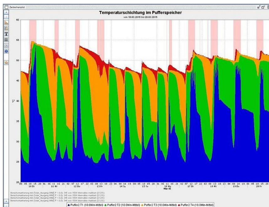
Figura 63: Stratificazione della temperatura nello stoccaggio termico monitorata da Monissoft (Fonte: Hochschule Rosenheim)
