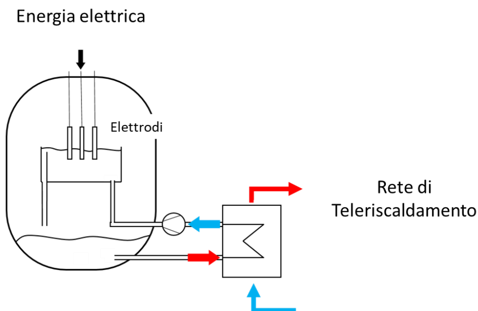
Figura 50: Schema di una caldaia a elettrodi (Fonte: AGFW)
