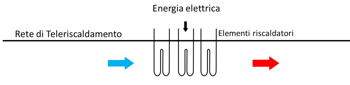
Figura 52: Schema di un riscaldatore di flusso elettrico (Fonte: AGFW)
