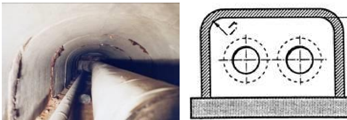
Figura 30: Condutture sotterranee, immagine di un canale rivestito (AGFW, 2013) (sinistra) e un canale rettangolare, come previsto dalla norma DIN 18178 (AGFW, 1993) (destra)
