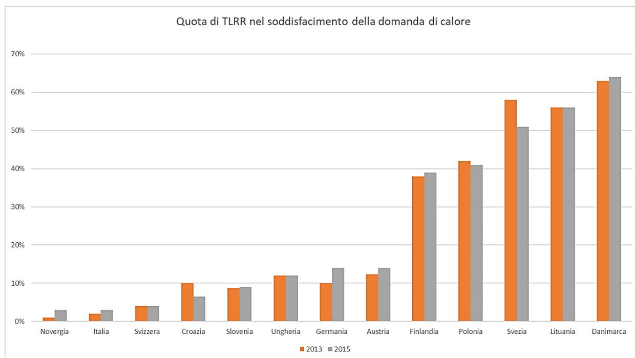
Figura 12: La quota di teleriscaldamento e teleraffrescamento rispetto ad altre soluzioni di riscaldamento in Europa (Fonte: Executive Summary by Gerdvila, Country by Country 2017, Euroheat & Power)
