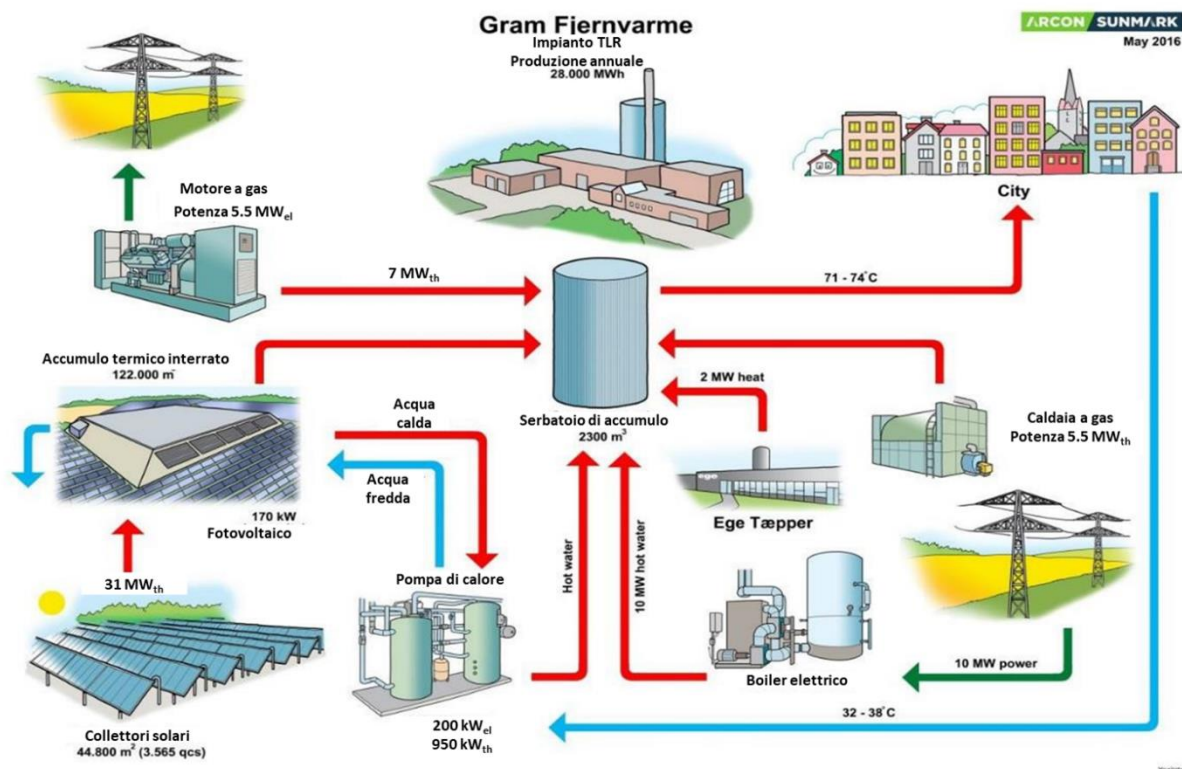
Figura 5 Il sistema di teleriscaldamento decentralizzato con varie fonti di calore di Gram, Danimarca (Fonte: http://www.gram-fjernvarme.dk )
