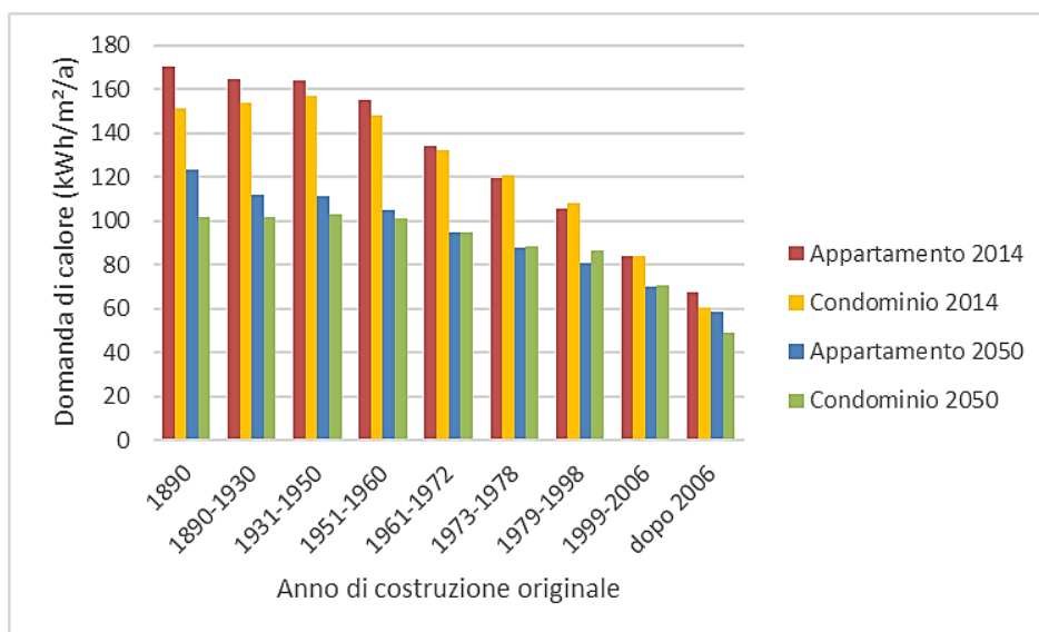
Figura 24: Potenziale di riduzione della domanda energetica 2050 (Fonte: Wittchen et al. 2014)
