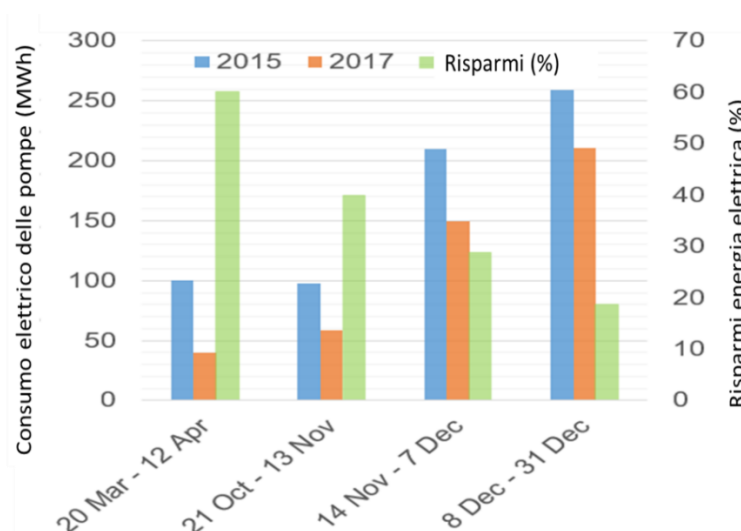
Figura 17: Domanda energetica per le operazioni di pompaggio nel 2015 e 2017 (Upgrade DH 2018b)
