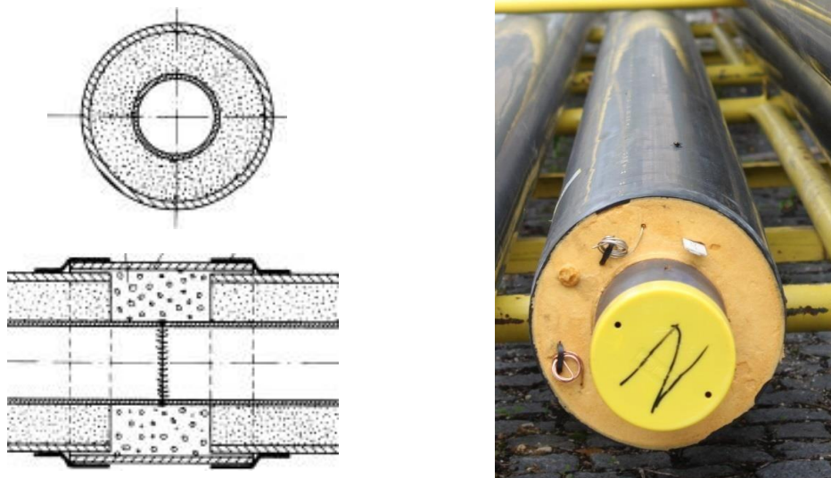
Figura 29: Sezione dei PJP e dei relativi collegamenti (Fonte: AGFW, 1993) (sinistra) e tubature (Fonte: D. Rutz) (destra)
