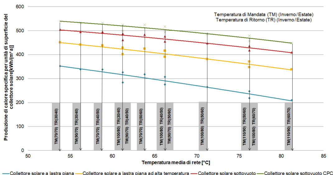
Figura 37: Resa di calore solare specifica per ogni area con collettori, rispetto alle temperature della rete di teleriscaldamento e per tipologia di collettori (dati atmosferici per la Germania meridionale) (Fonte: Solites)
