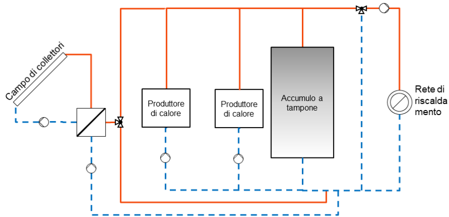
Figura 39: Collegamento in parallelo dei collettori solari termici alla rete di teleriscaldamento e teleraffreddamento per aumentare il flusso di ritorno della rete (Fonte: SOLITES)
