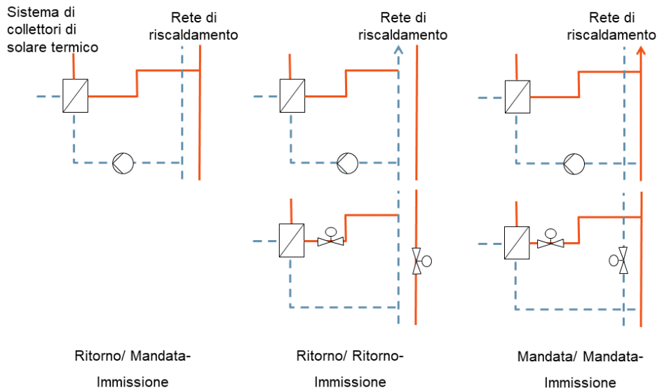
Figura 40: Tre concetti di alimentazione decentrata di calore solare nei sistemi di teleriscaldamento, con una pompa (parte superiore) o con valvole regolabili (parte inferiore) (Fonte: SOLITES)
