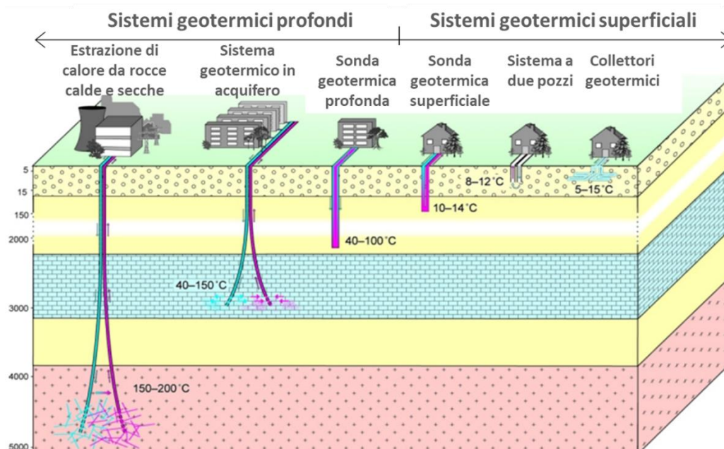
Figura 45: Diversi utilizzi dell'energia geotermica (sulla base di: Bayerisches Landesamt für Umwelt, 2016)
