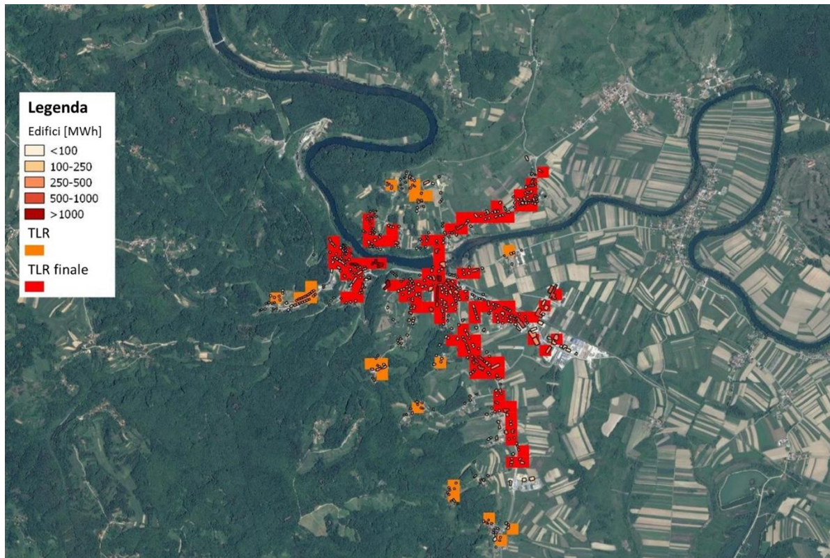
Figura 14. Mappa della domanda di calore nella città di Ozalj in Croazia, che mostra anche le parti della città in cui sarebbe possibile effettuare il collegamento con un sistema di teleriscaldamento (parti arancioni e rosse) (Fonte: Doračić et al. 2018)
