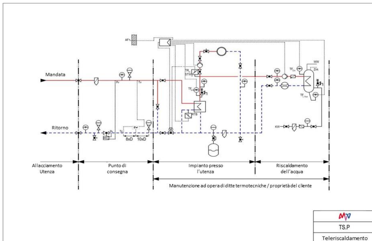
Figura 8: Lo schema di un sistema indiretto (Fonte: MVV Netze, 2015)
