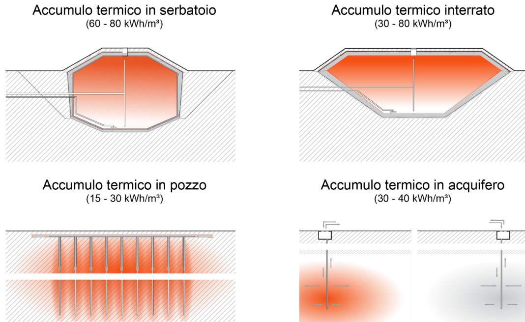
Figura 56: Panoramica dei concetti di stoccaggio dell'energia termica sotterraneo (Fonti: Solites)
