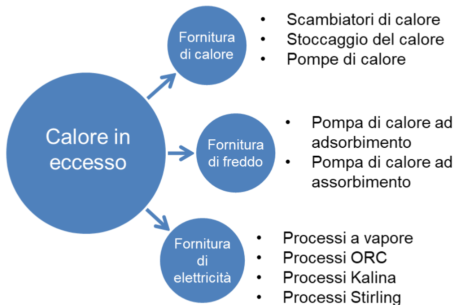
Figura 48: Utilizzo del calore in eccesso e attrezzatura utile (Secondo Hirzel et. al., 2013)
